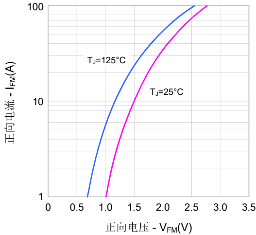
图15. 正向特性
