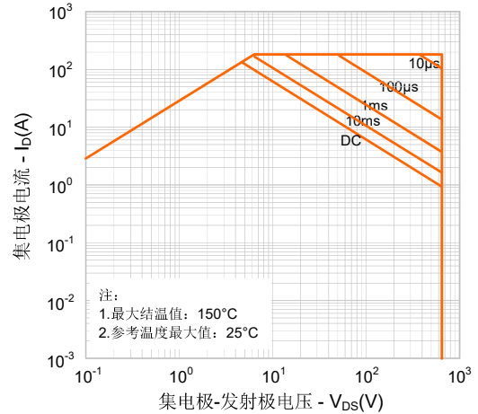
图18. 最大安全工作区域
