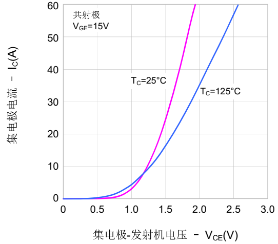
图2. 典型饱和和降压特性
