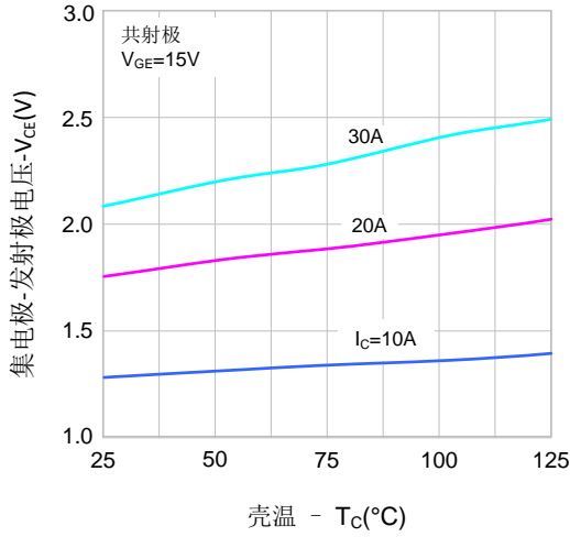
图6. 饱和电压 vs. 温度
