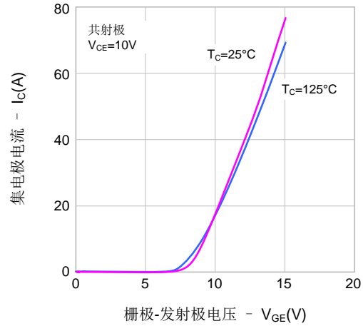
图3. 传输特性
