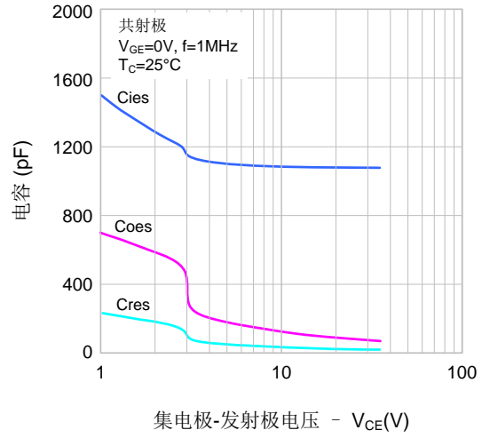
图7. 电容特性
