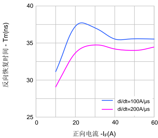
图16. 反向恢复时间 vs. 正向电流
