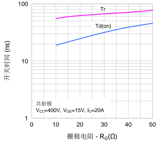
图9. 导通特性 vs. 栅极电阻
